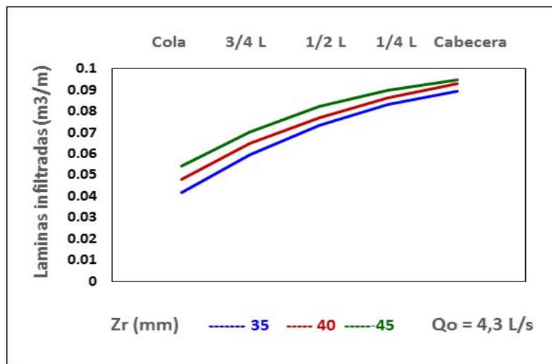
Figura 5. Láminas infiltradas en función de los tiempos de oportunidad
