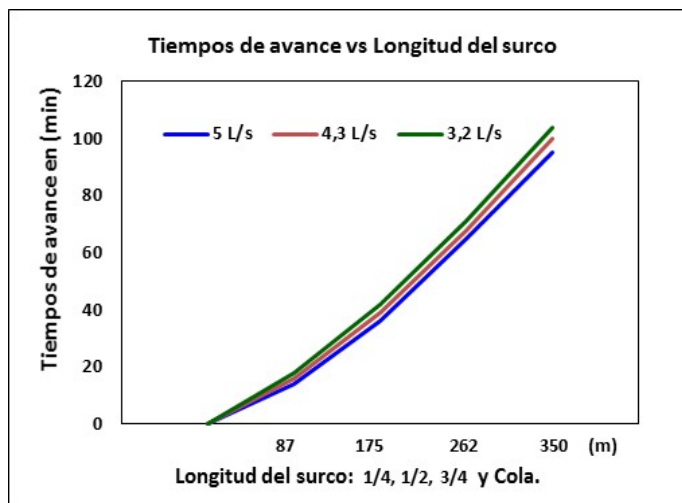
Figura 3. Curvas de avance para los 3 caudales evaluados
