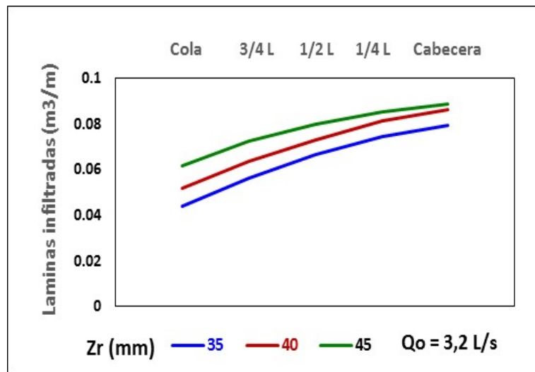
Figura 4. Láminas infiltradas en función de los tiempos de oportunidad
