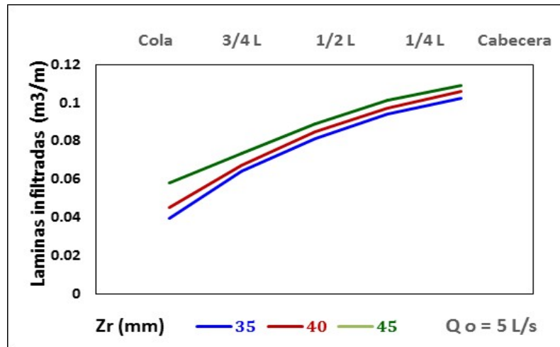
Figura 6. Láminas infiltradas en función de los tiempos de oportunidad
