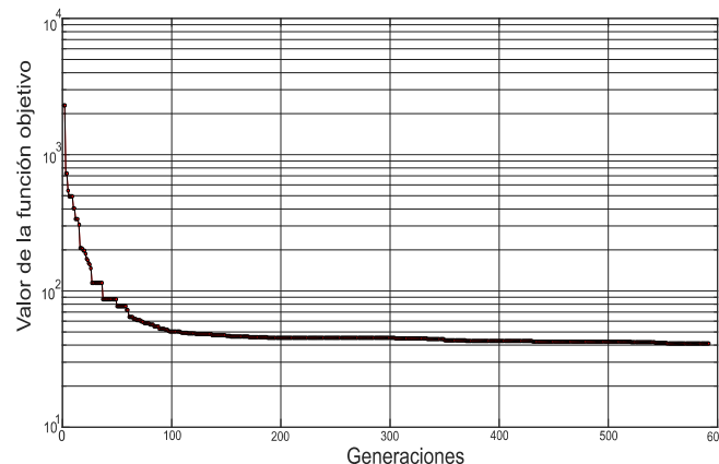
Figura 9. Comportamiento típico del algoritmo DE en las ejecuciones de la calibración del modelo SCC
