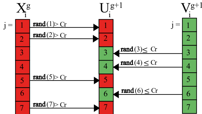
Figura 2. Representación de un posible esquema de cruzamiento para el caso D = 7 . (Modificada de Storn y Price 1997)
