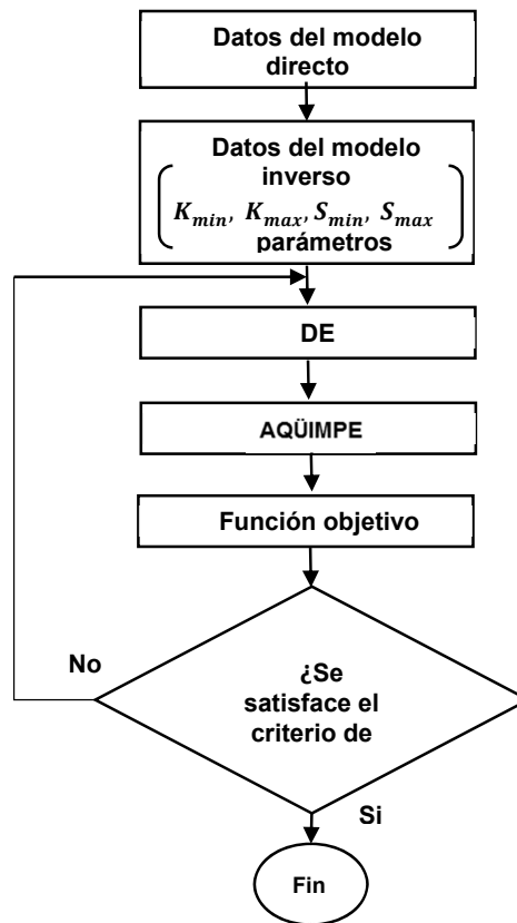
Figura 3. Diagrama de flujo de la herramienta META - AQÜIMPE con el algoritmo evolución diferencial acoplado
