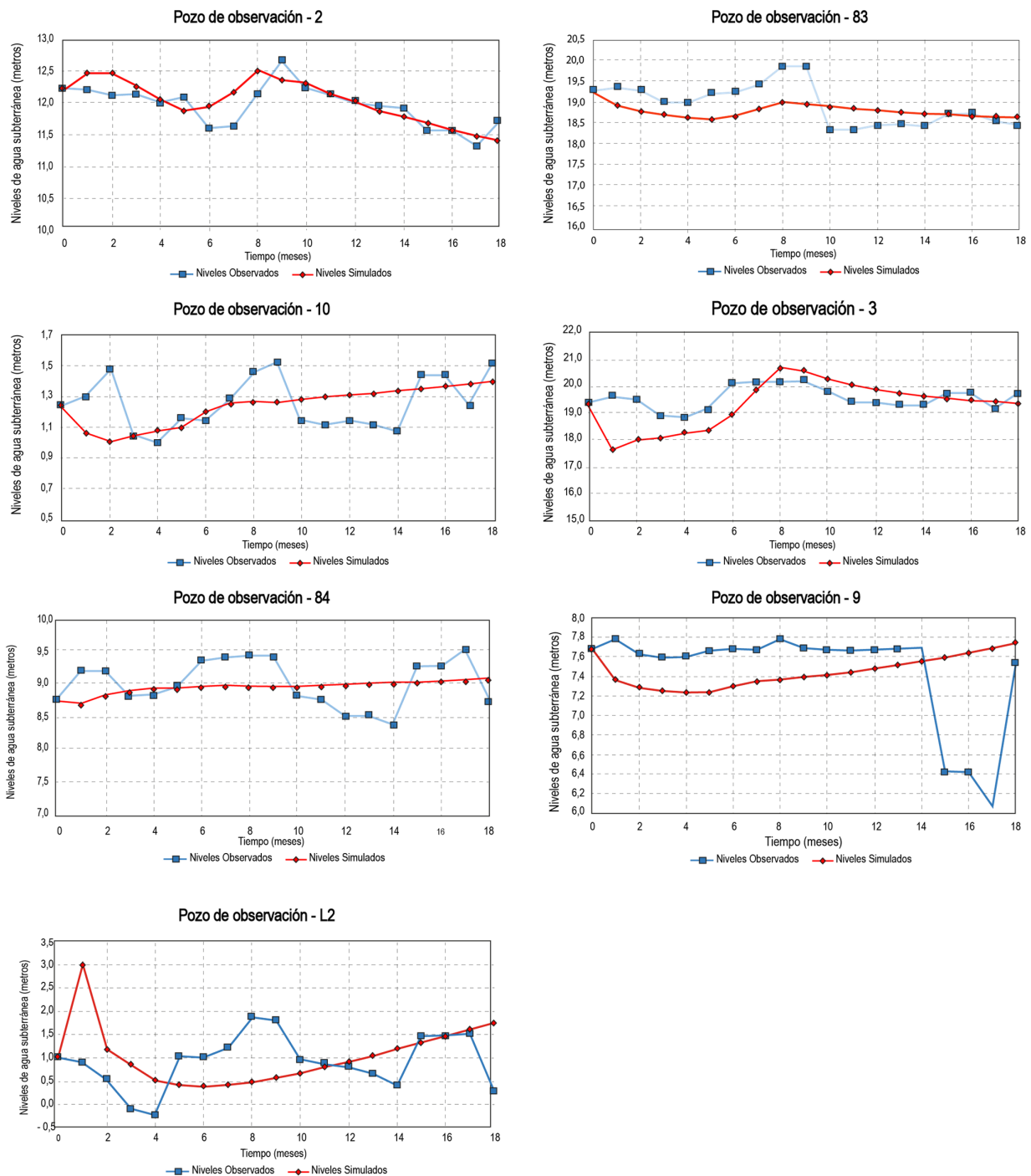
Figura 10. Niveles observados y simulados en el período de calibración
