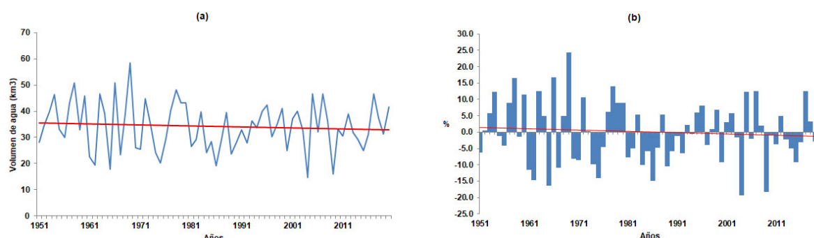
Figura 6. (a) Esguerrimiento anual estimado por Budyko y (b) Anomalía del esguerrimiento anual respecto a la línea base 1961-1990
