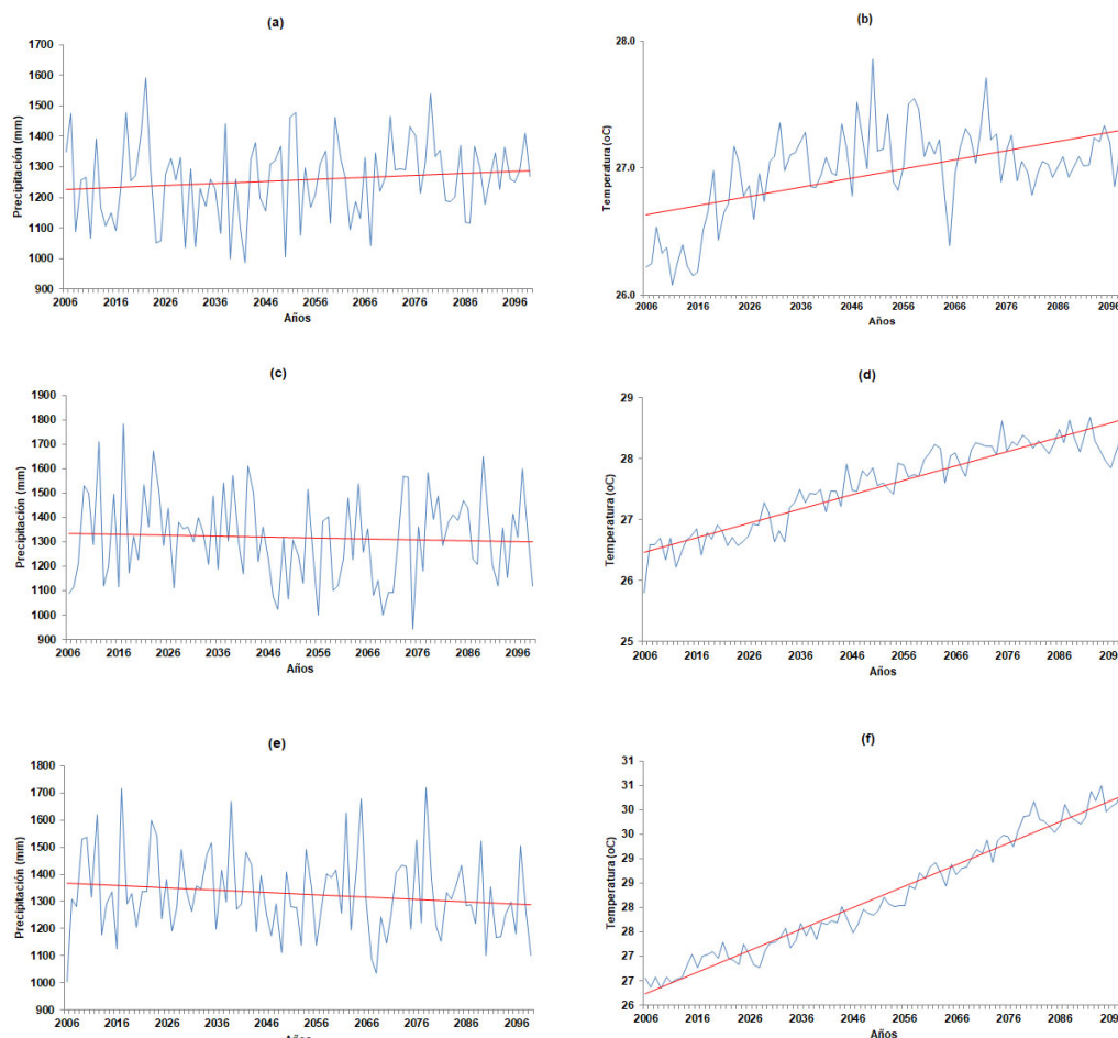
Figura 7. Precipitación anual (mm) y temperatura anual promedio del aire (°C): (a) Precipitación RCP 2.6, (b) Temperatura RCP 2,6; (c) Precipitación RCP 4,5; (d) Temperatura RCP 4,5; (e) Precipitación RCP 8,5; (f) Temperatura RCP 8,5. Fuente: CITMA, 2020
