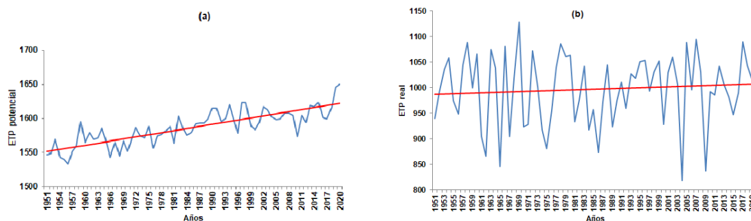
Figura 2. (a) Evaporación potencial a la izquierda y (b) Evaporación real a la derecha. Estimadas por modelo de Budyko (Rivero, 2008)
