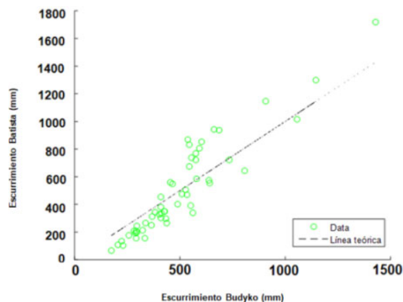
Figura 4. Relación entre esguerrimientos estimados por Budyko y observado en estaciones hidrométricas. Coeficiente de correlación r=0.93 . Período 1964-1988
