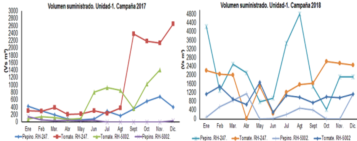
Figura 6. Volumen de agua suministrado a los cultivos de pepino y tomate, unidad 1.
