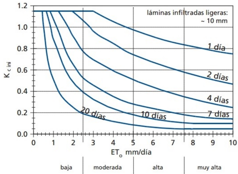
Figura 4. K_{c\ ini} Para todo tipo de suelo con láminas de (3-10mm por evento). Allen et al. 1998.
