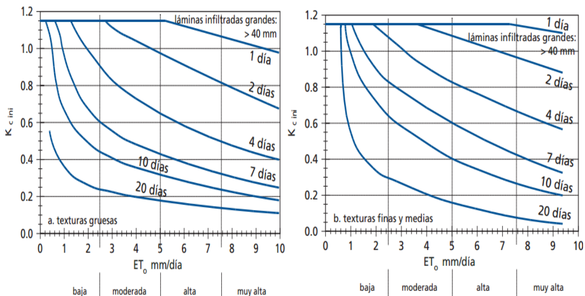
Figura 5. K_{c\ ini} relacionado con el nivel de ET_0 y el intervalo entre riegos con láminas \geq 40 mm. Allen et al. 1998.
