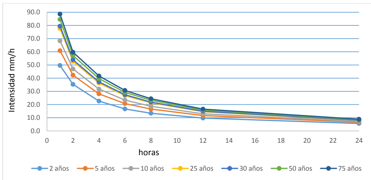
Figura 4. Curvas de intensidad, duración y frecuencia para diferentes períodos de retorno
