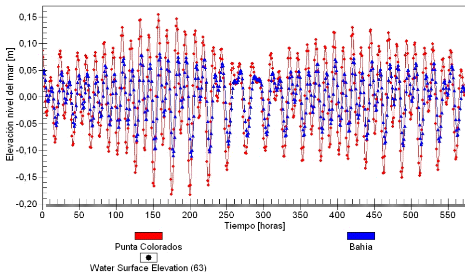
Figura 3. Comportamiento de la señal que entra en la bahía y aquella que se registra en Cayo Loco
