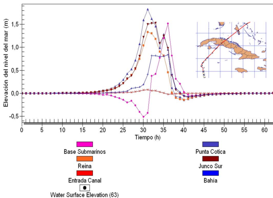
Figura 5. Variación de la altura máxima del agua en los puntos de observación al paso del huracán Michelle, 4 nov. 2001
