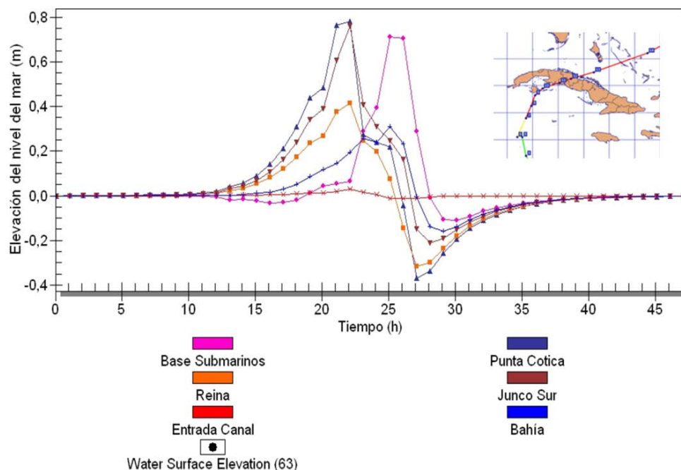
Figura 4. Variación de la altura máxima del agua en los puntos de observación al paso del huracán Lili, 18 Oct. 1996
