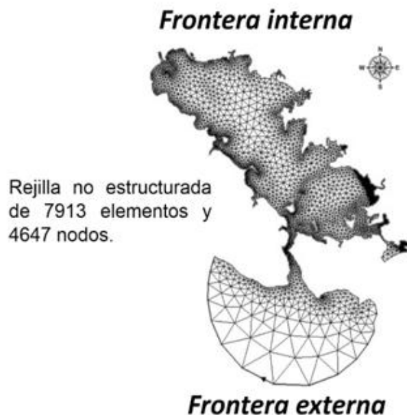
Figura 2. Dominio computacional utilizado
