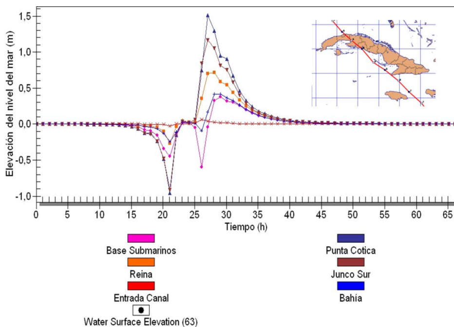
Figura 6. Variación de la altura máxima del agua en los puntos de observación al paso del huracán Dennis, julio 2005
