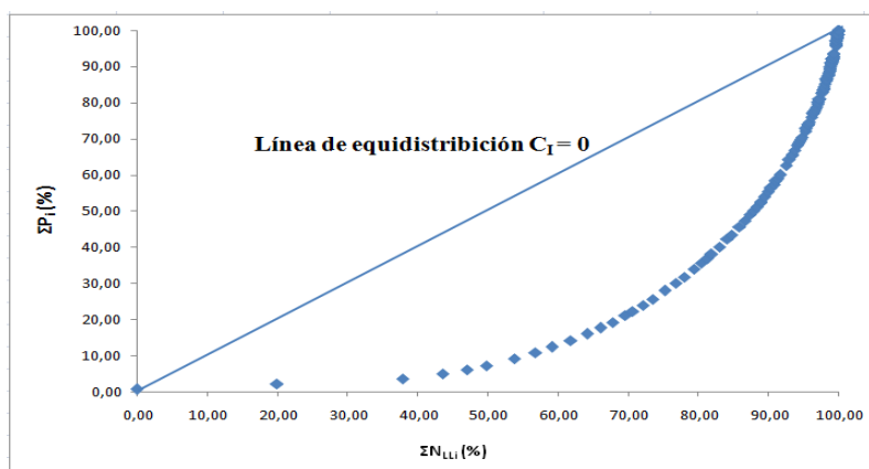
Figura 3. Curva de ajuste
