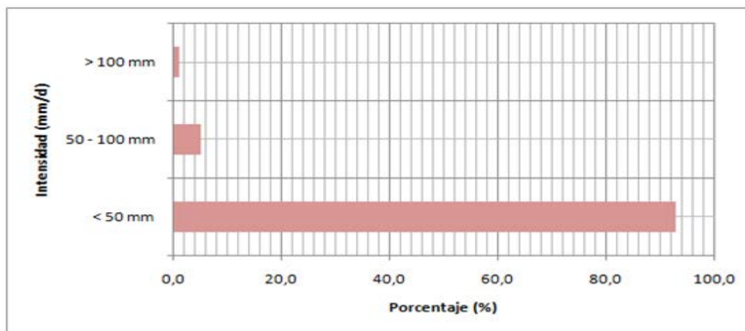
Figura 5. Distribución de las precipitaciones en tres intervalos de intensidades
