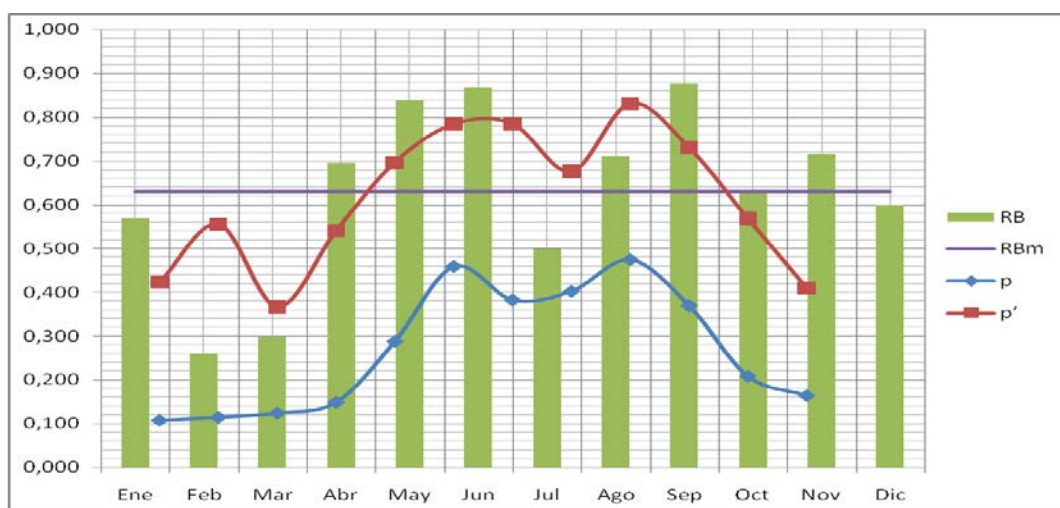
Figura 8. Probabilidades y coeficiente de persistencia de la lluvia
