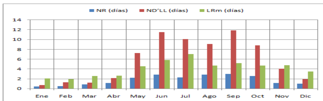
Figura 7. Número y longitud media de rachas; número de días con precipitaciones después de haber llovido
