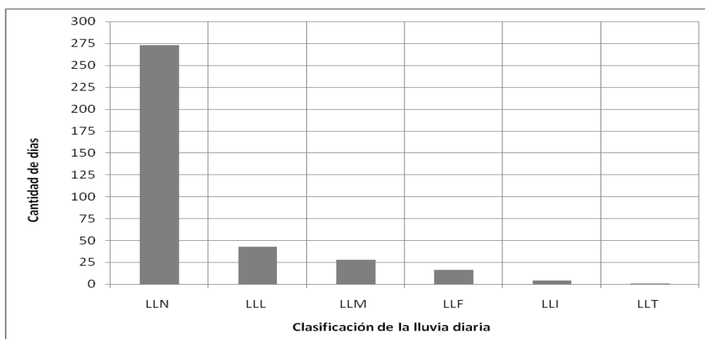
Figura 4. Distribución de las lluvias diarias según el rango de agrupación
