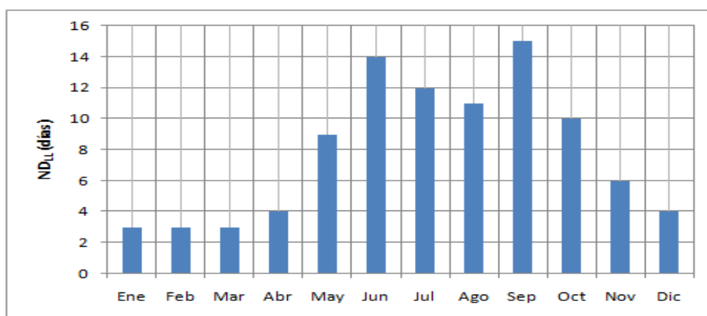
Figura 6. Número de días con lluvias por mes en el periodo 1983-2012
