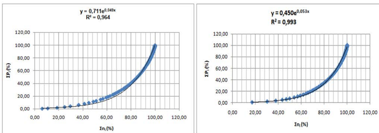
Figura 10. Curva exponencial de la lluvia diaria en los pluviómetros CA-722 y CA-894
