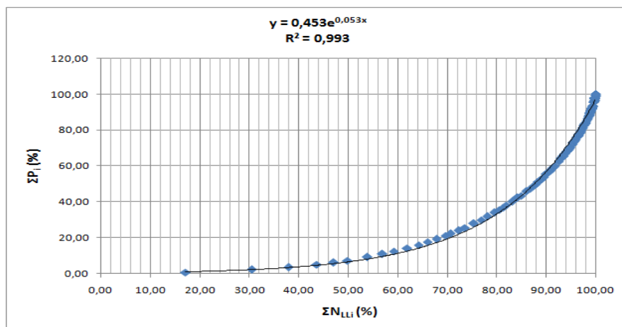
Figura 11. Curva exponencial de la lluvia diaria en Ciego de Ávila
