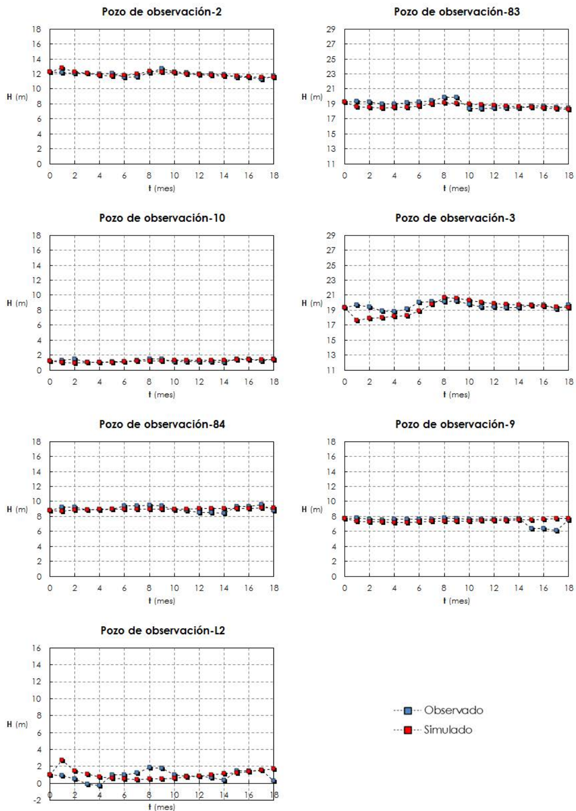
Figura 10. Niveles observados y simulados en el período de calibración
