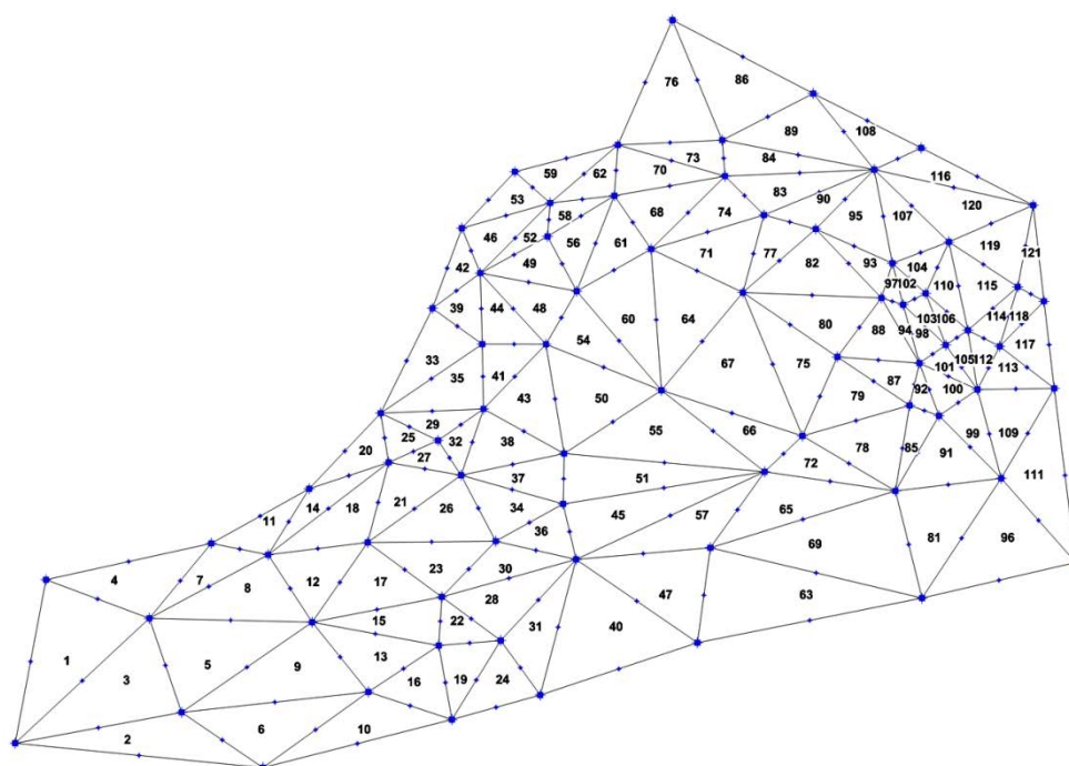
Figura 7. Discretización en el sector Cuentas Claras
