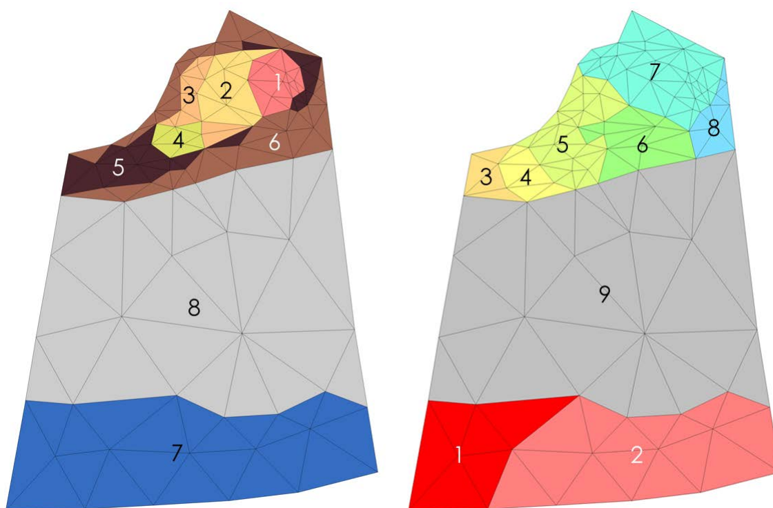
Figura 5. Grupos de Propiedades (izquierda) y Grupos de Infiltración (derecha).
