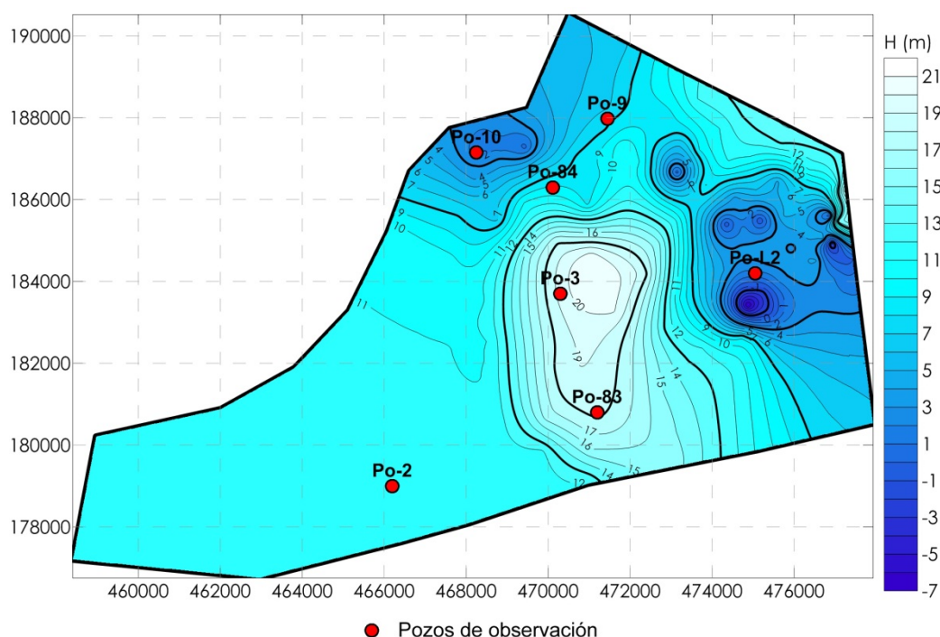
Figura 11. Mapa de hidroisohipsas correspondiente al tiempo final de la calibración
