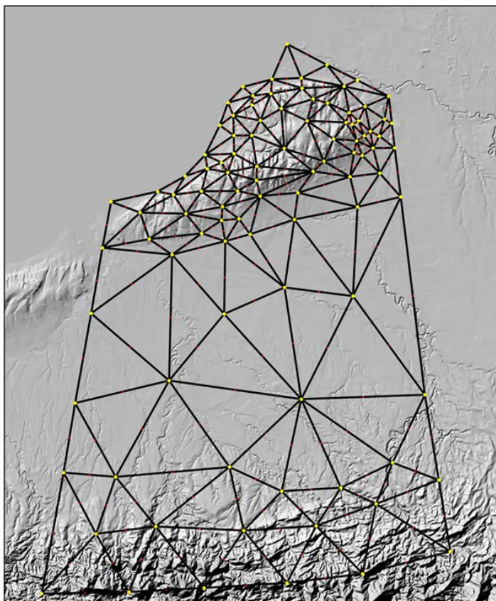
Figura 4. Discretización del área de Cuentas Claras (área total)
